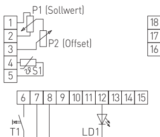
Anschlussbild
