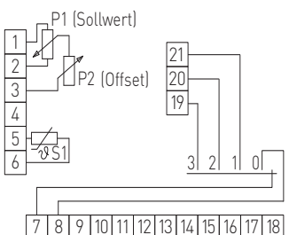
Anschlussbild
